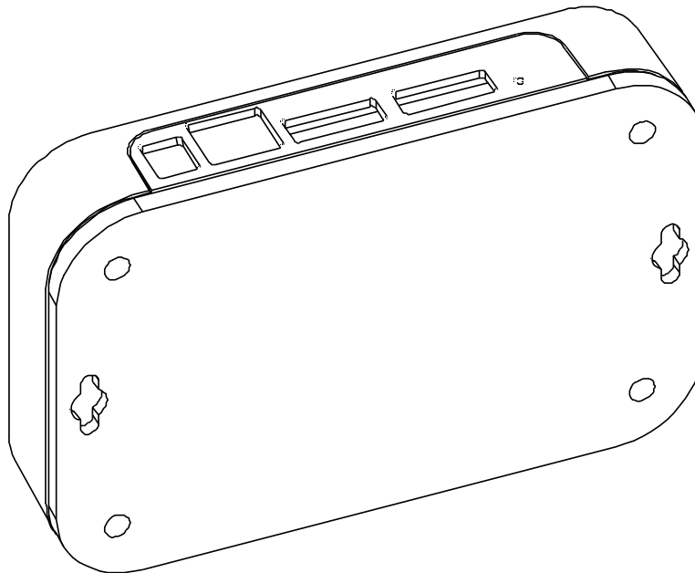
Rys.2. Rozmieszczenie otworów montażowych
